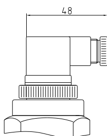
DIN 43650 A
