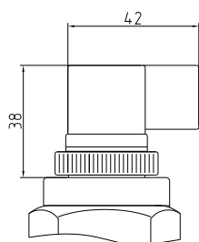
DIN 1/2" FEMALE
